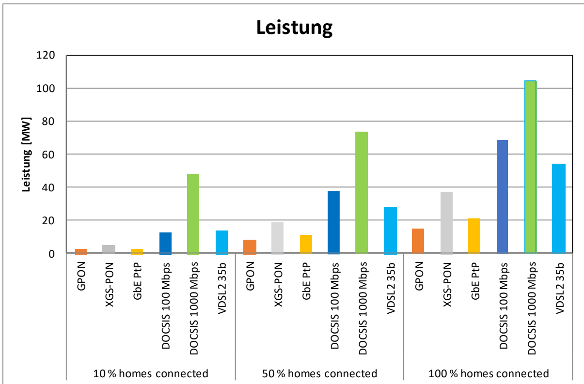
ABBILDUNG 18: LEISTUNGS-AUFNAHME FÜR EINE VERSORGUNG DER LÄNDLICHEN GEBIETE IN DEUTSCHLAND MIT DER JEWEILIGEN ZUGANGSNETZTECHNOLOGIE FÜR VERSCHIEDENEN AUSLASTUNGSGRADU (ANTEIL HOMES CONNECTED).
