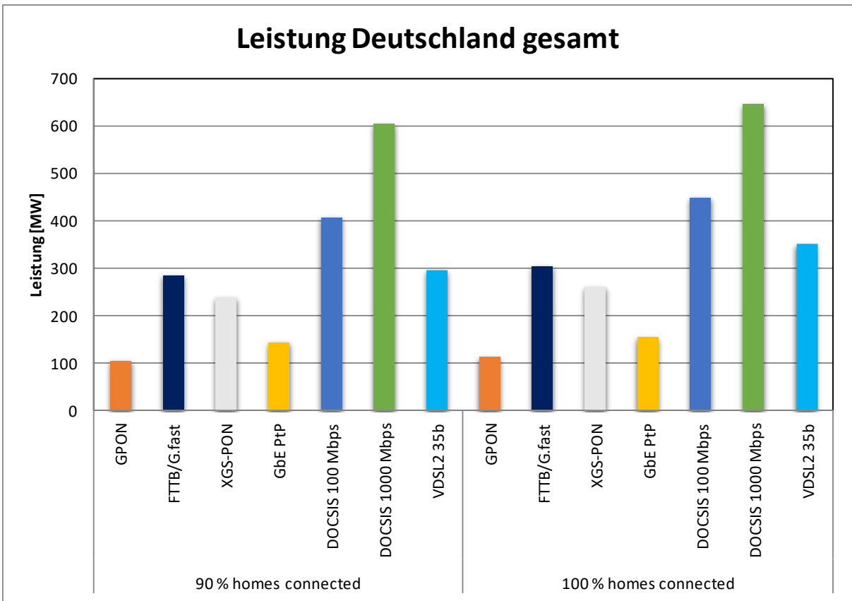
ABBILDUNG 10: LEISTUNGS-AUFNAHME FÜR EINE GESAMTVERSORUNG VON DEUTSCHLAND MIT DER JEWEILIGEN ZUGANGSNETZTECHNOLOGIE FÜR VERSCHIEDENEN AUSLASTUNGSGRAD (ANTEIL HOMES CONNECTED).
