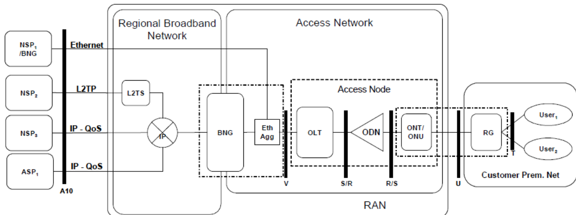
ABBILDUNG 4: NETZARCHITEKTUR FÜR EHTERNET-BASIERTE GPON BREITBAND-ZUGANGSNETZE. QUELLE: [13]
